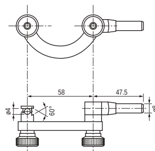
2349999 Supporto di centraggio
